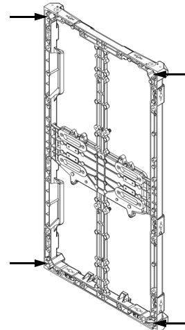
Avant Trous de fixation taille M10 (x4)
